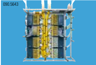
Оптические кроссы высокой плотности - ODF
